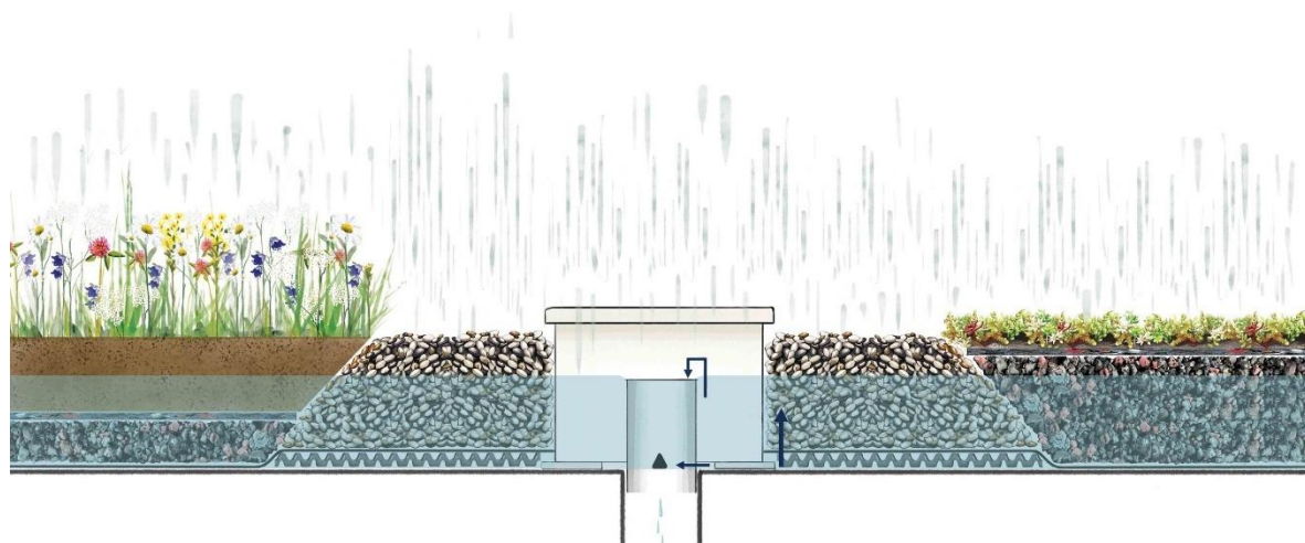
Figur 2.3. Illustrasjonen er hentet fra www.bergknapp.no og viser oppbygningen av et blågrønt tak med restriktor i midten, semi-intensivt tak med engvegetasjon til venstre og ekstensivt tak med sedummatter lengst til høyre.
